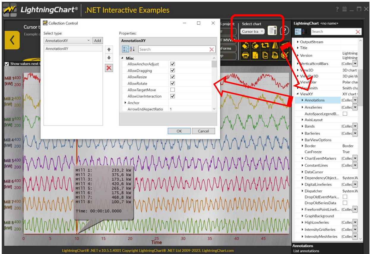
图 5-8. LightningChart 的对象模型。即时编辑 AnnotationXY 属性
