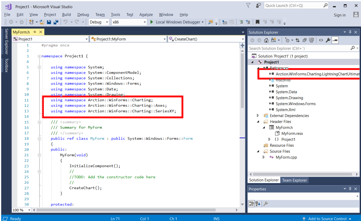
图 27-5. 将 Arction.WinForms.Charting.LightningChart.dll 包含在引用列表中，并在项目中添加相关命名空间。在版本 11.0+ 中，参考是 LightningChart.WinForms.Charting.NET4。
