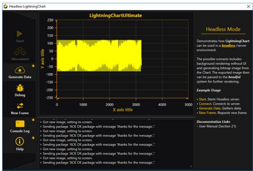
图 254-2. WPF 客户端 app; 启动、连接、生成数据后, 会显示连续更新的图像流。
