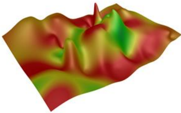
图 7-38. PalettedByValue.
