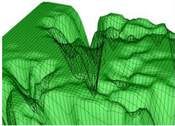
图 7-48. DrawWireframeThrough 开启.
