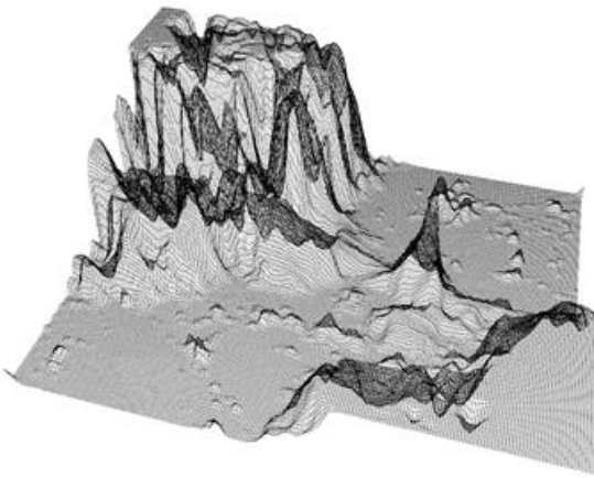
图 7-40. WireframeType = Wireframe.
