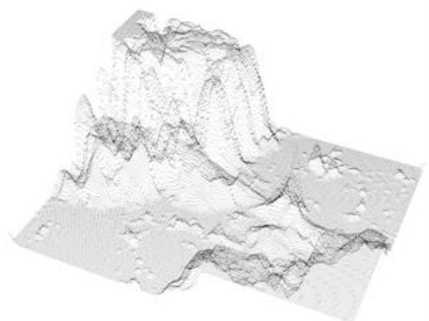
图 7-43. WireframeType = Dots.
