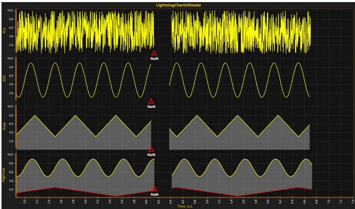
图 6-96. DataBreaking 用于 PointLineSeries、SampleDataSeries、AreaSeries 和 HighLowSeries.
