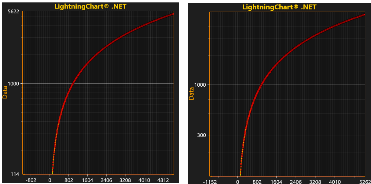
图 6-31。在左侧图表的 X 轴上 PreferEndPointLabelsOverNearbyMajorTick 被禁用，而在右侧这个属性是启用。左侧图表的 Y 轴设置为始终显示结束标签（ EndPointLabelsVisible=true ， EndPointMajorTickThreshold=-1 ），而右侧图表的 Y 轴配置为除了一个主要刻度外还显示一个次要刻度（ EndPointLabelsVisible=true ， EndPointMajorTickThreshold=1 ）
