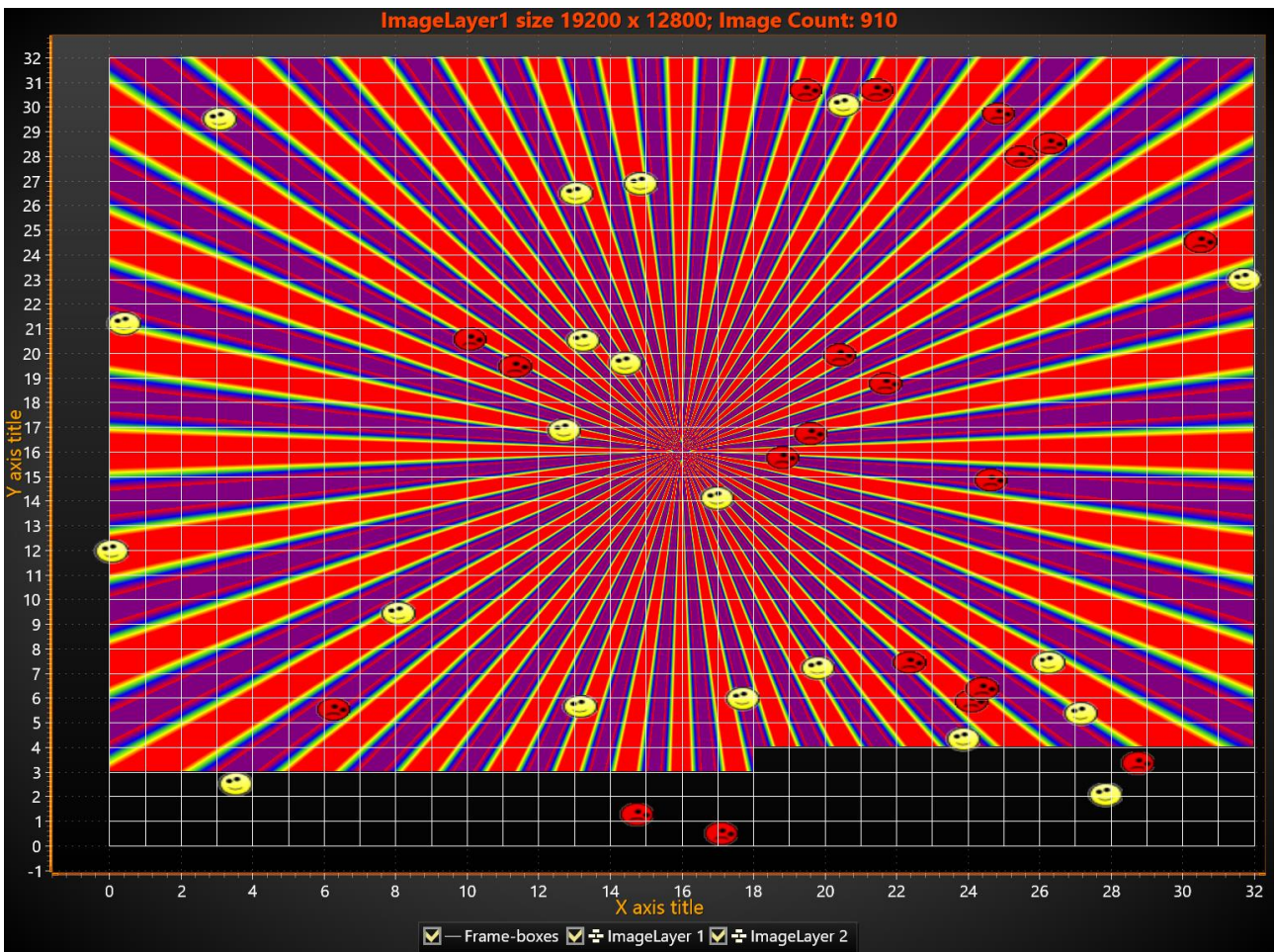
图 6 136. 两个 ImageLayers 正在使用中，其中一个仍在加载中
