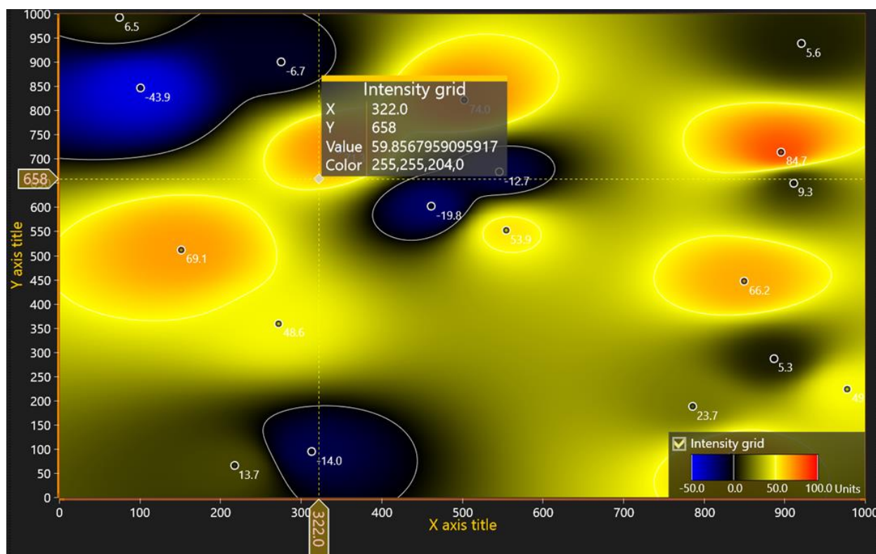
Figure 6-124. 数据光标跟踪强度网格。除了 X 和 Y 值外，光标还显示网格的值和颜色字段
