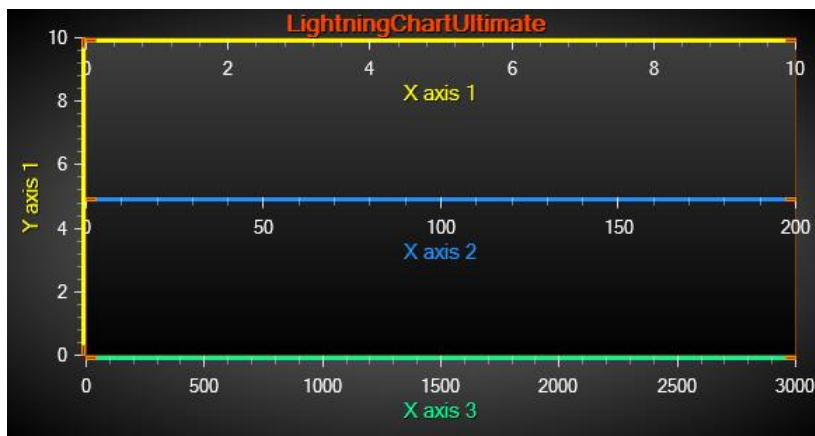
图 6-9. XAxisAutoPlacement = Off ; 禁用自动布置轴，每个轴的位置（Position）和对齐（Alignment）属性各自分别应用。 第一条轴 Position = 0 ，第二条轴 Position = 50 ，第三条轴 Position = 100
