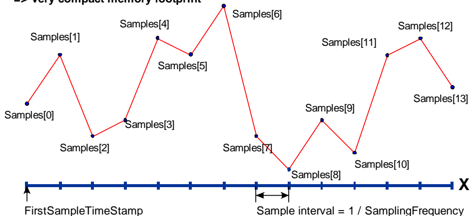
图 6-42. SampleDataSeries 概览
