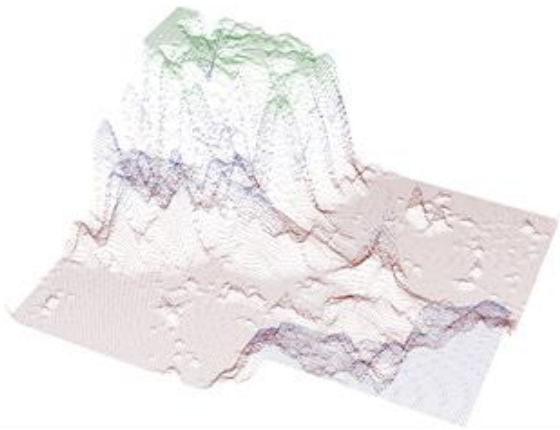
图 7-44. WireframeType = DotsPalettedByY.
