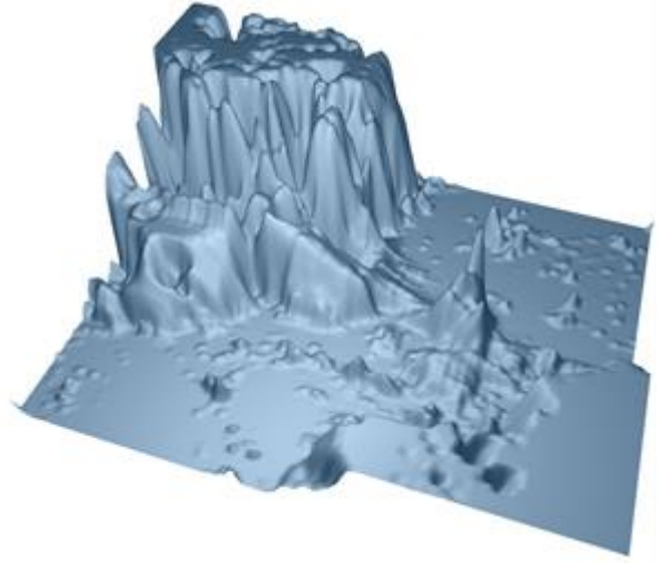
图 7-35. Toned 填充.
