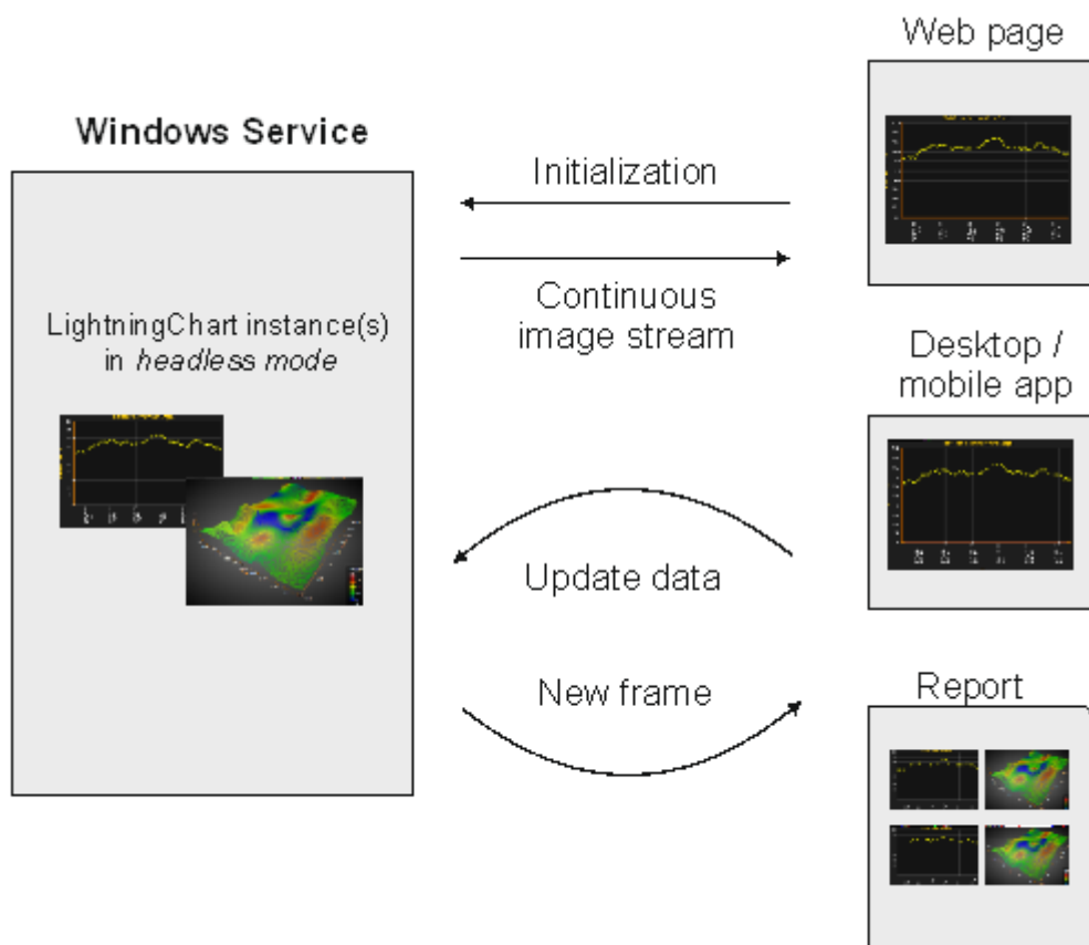
图 254-1. 示例用法图解.
