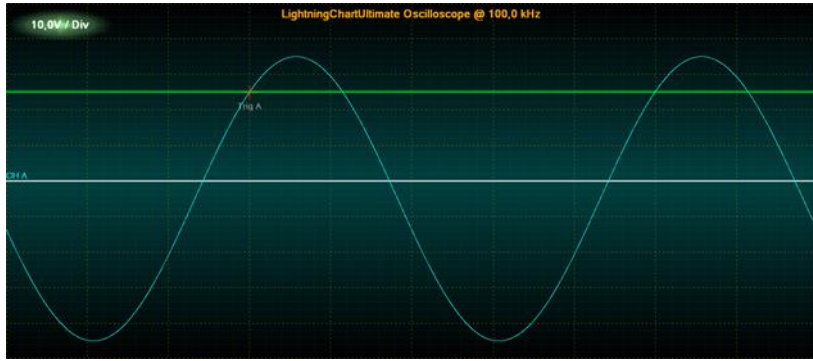
图 199-2. 采用如上设置的一种简单的正弦波形信号
