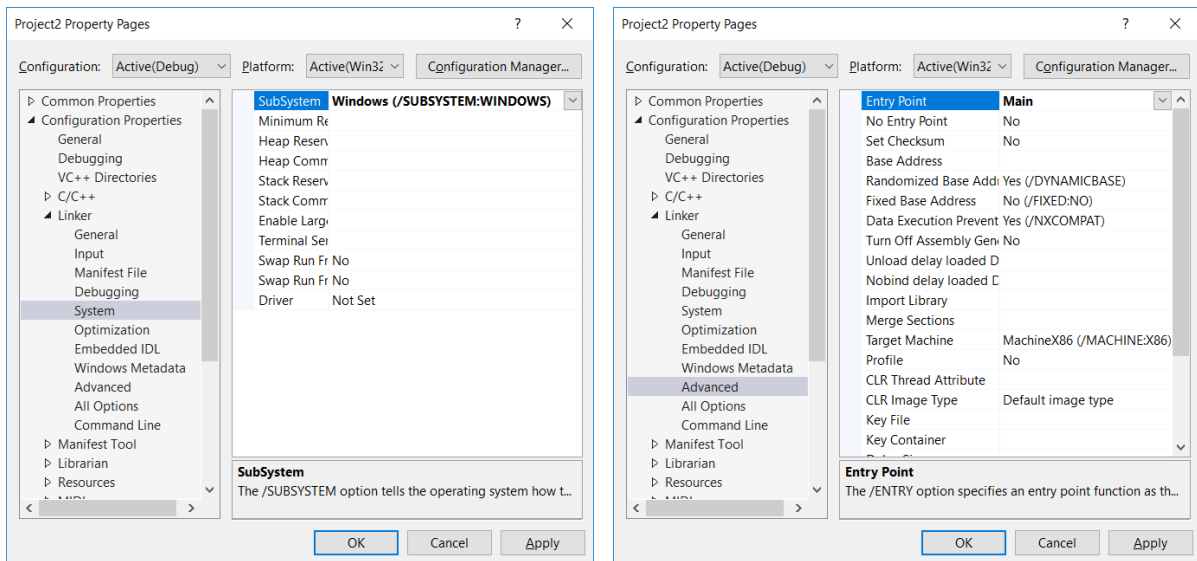
图 27-3. C++项目属性页
