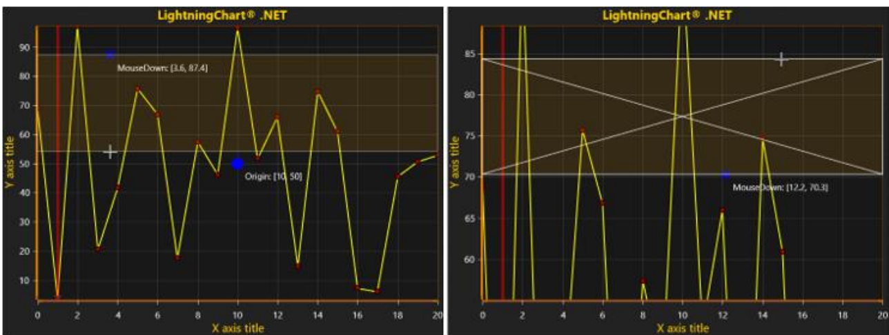
图 6-92. ZoomPanOptions.RectangleZoomMode = Vertical . 只对 Y 轴缩放，X 轴保持不变。
