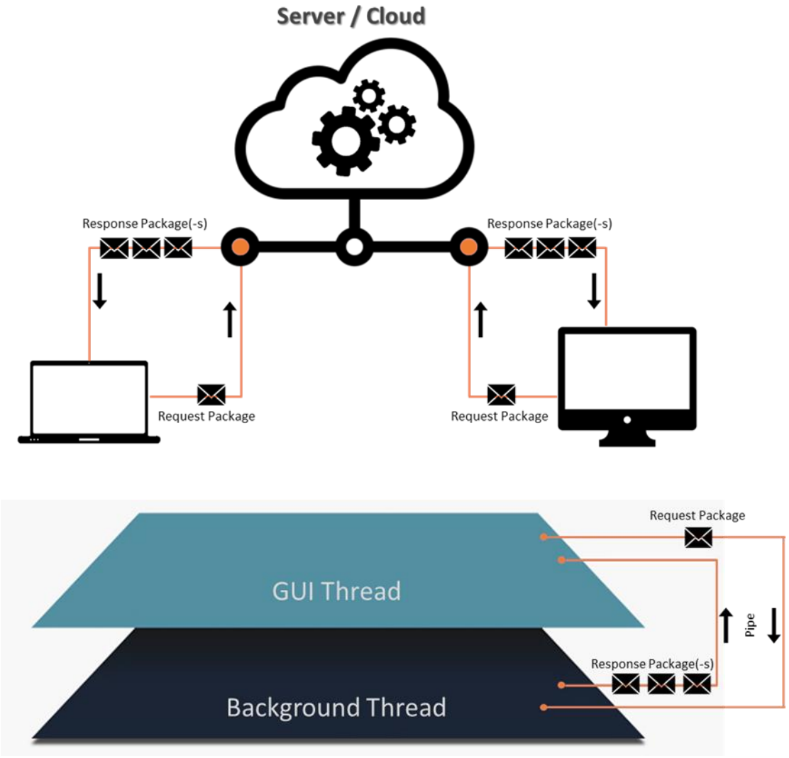
图 254-3. 无头演示服务——消息的客户端内部操作, 带有图示说明的命名管道和后台线程。
